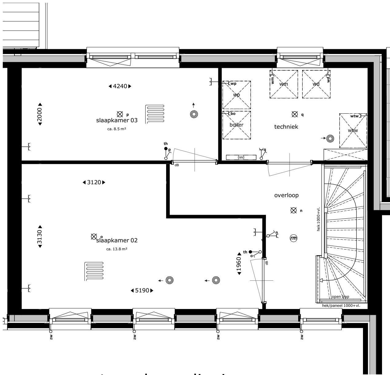
tweede verdieping
