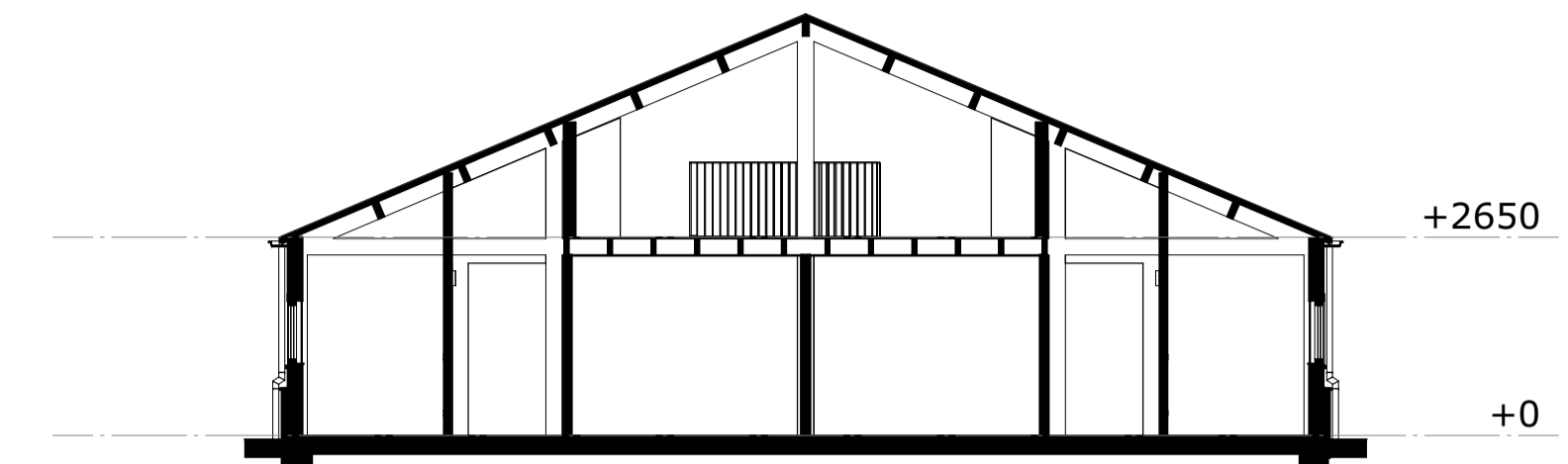
doorsnede A
