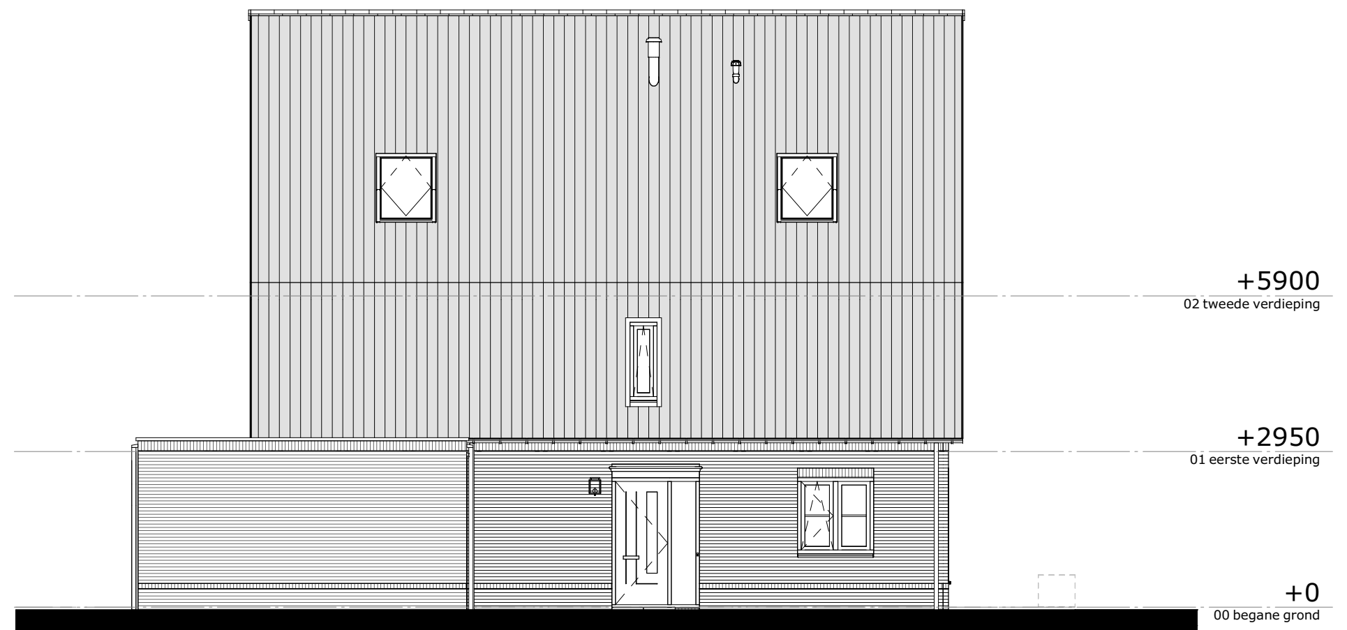
linker zijgevel
