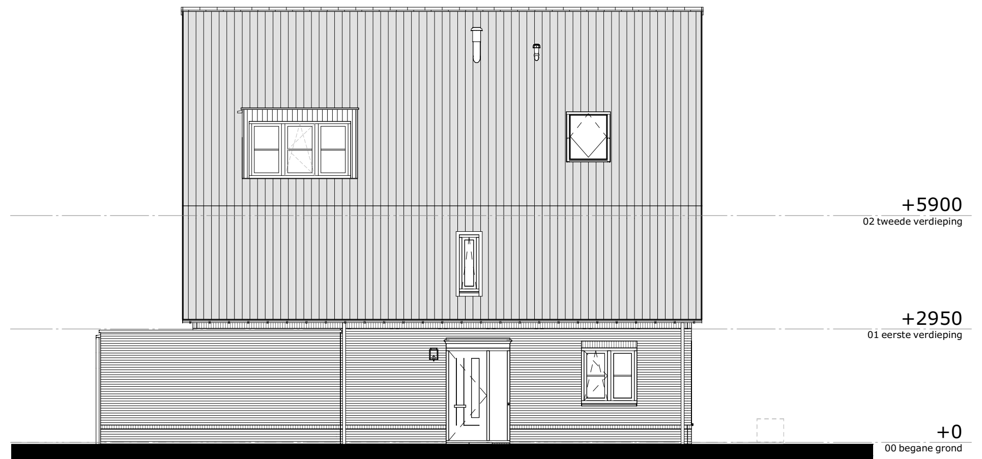
Dakkapel: getekend : bwnr 38 linker zijgevel
