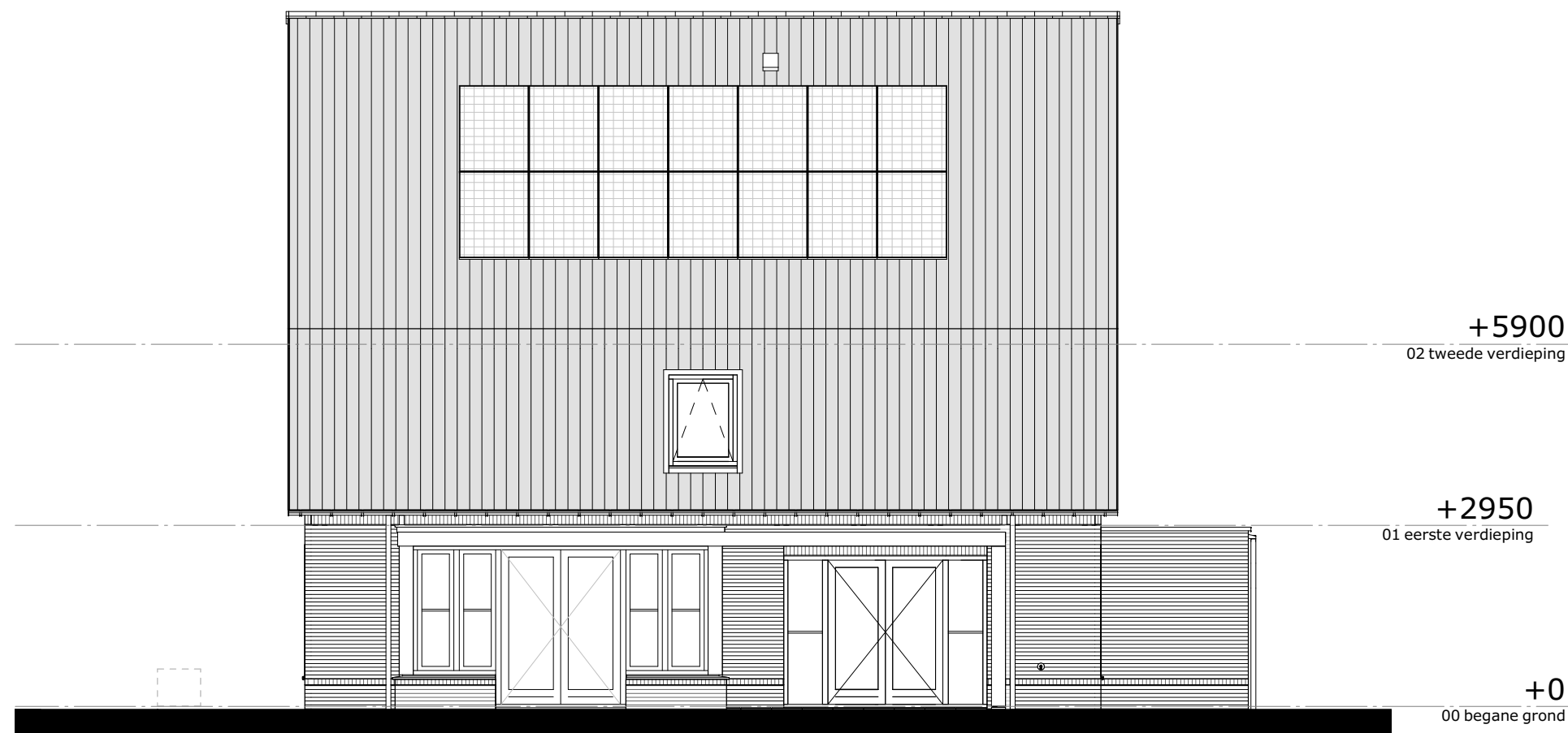
Erker zijgevel: getekend : bwnr 38 rechter zijgevel
