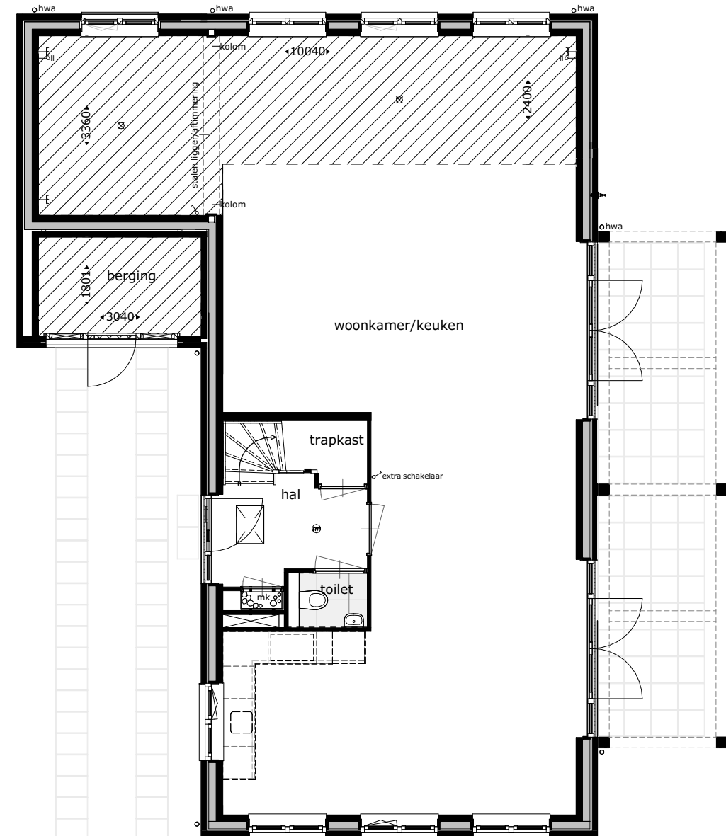
begane grond: optie 00032
