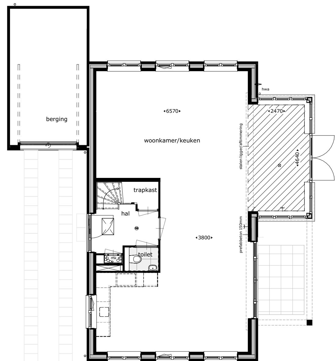
Erker zijgevel: getekend : bwnr 38 begane grond: optie 00042
