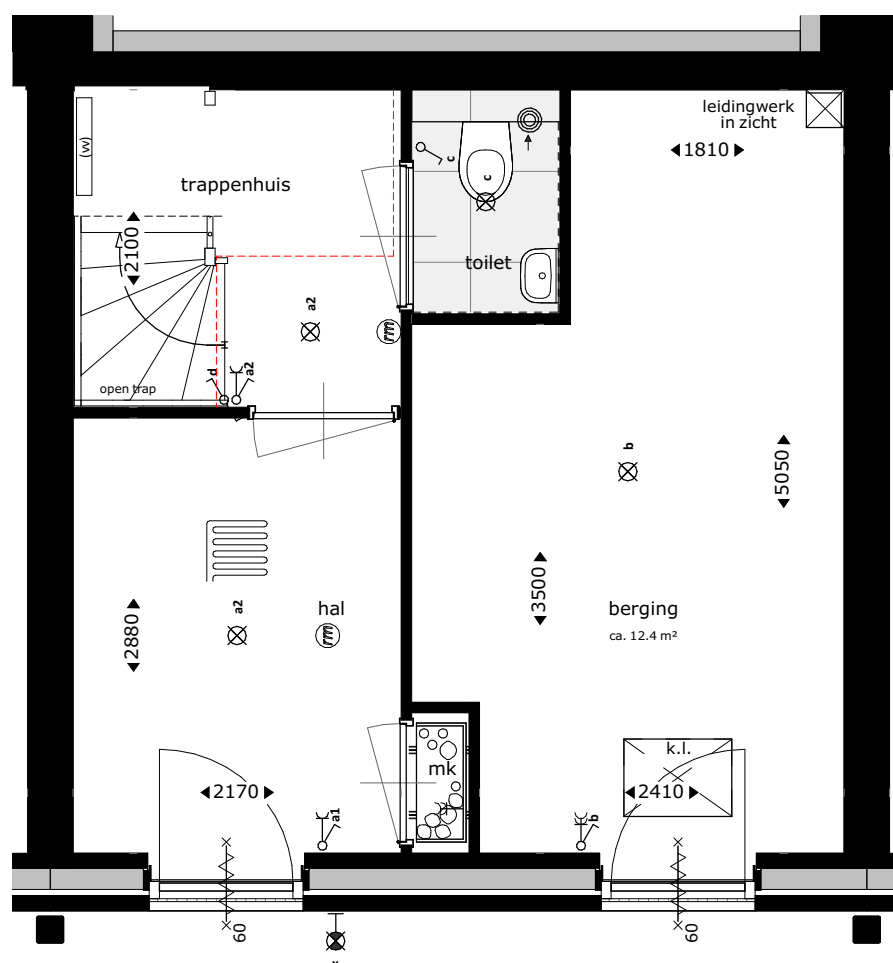
parkeerniveau
