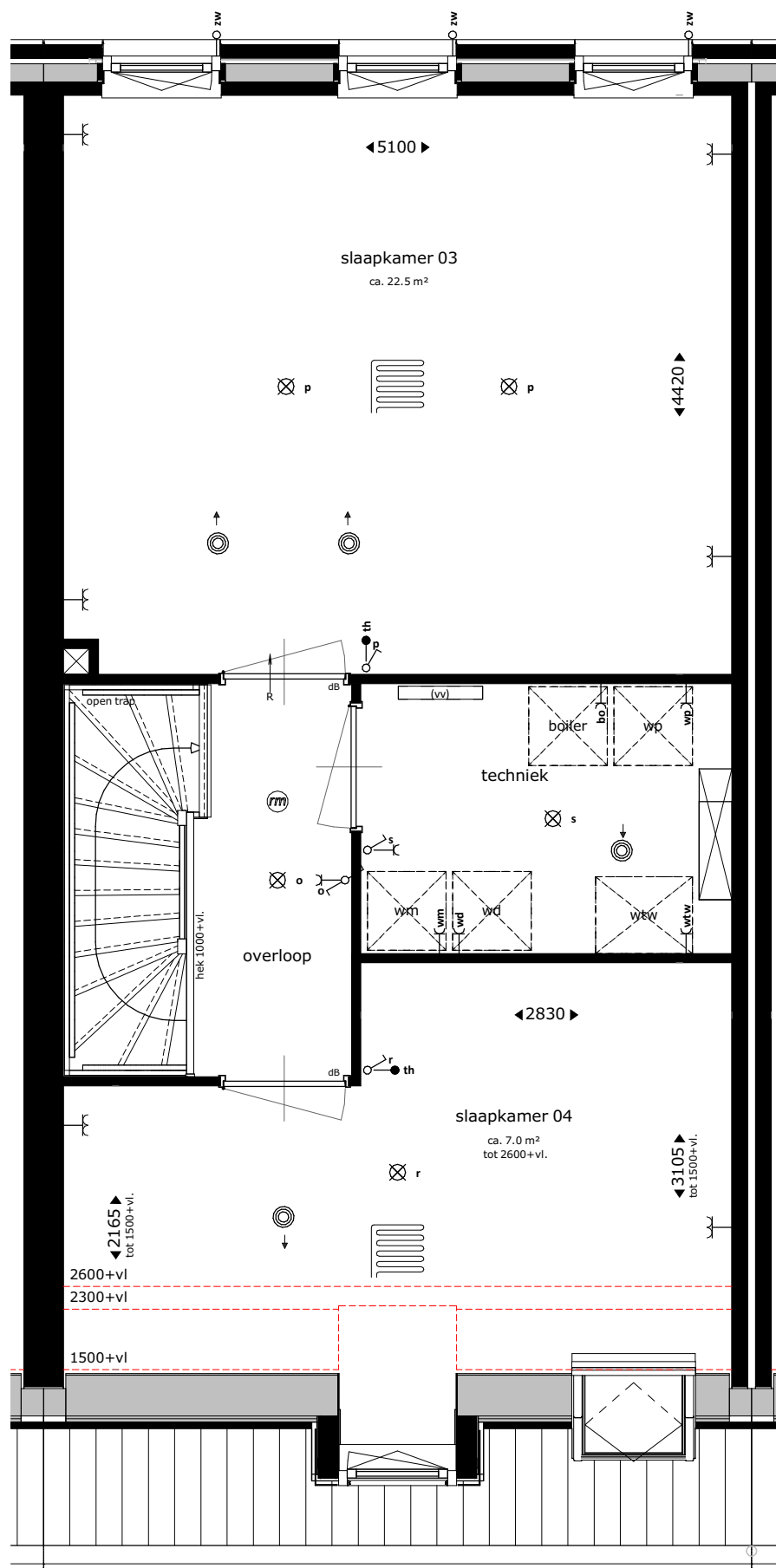
tweede verdieping
