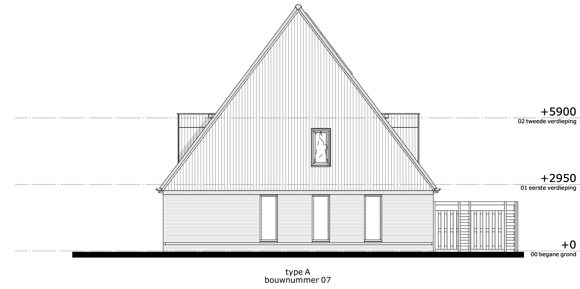
rechter zijgevel
