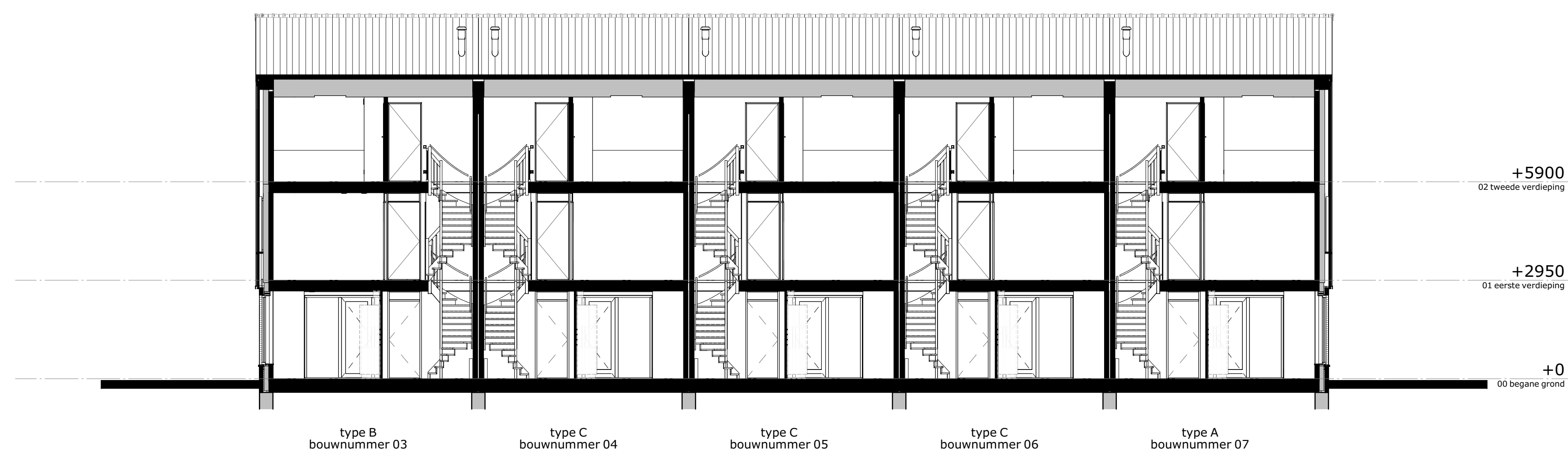
doorsnede B
