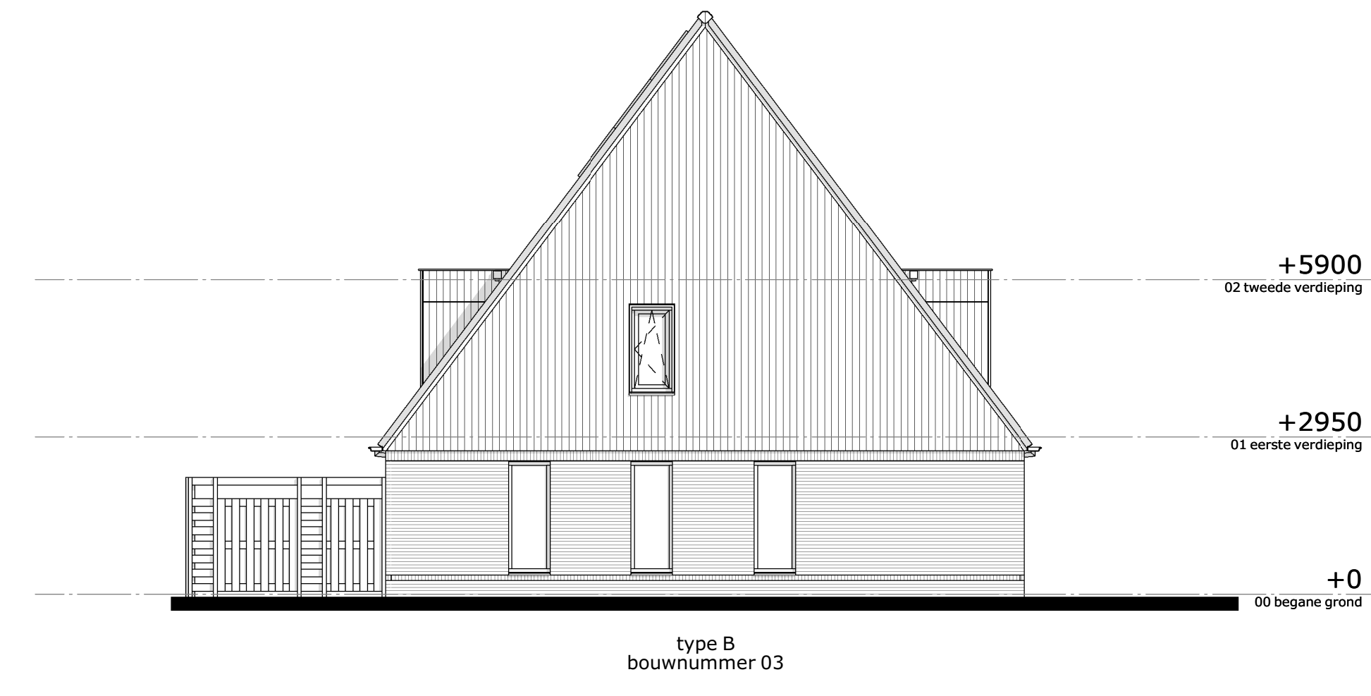
linker zijgevel
