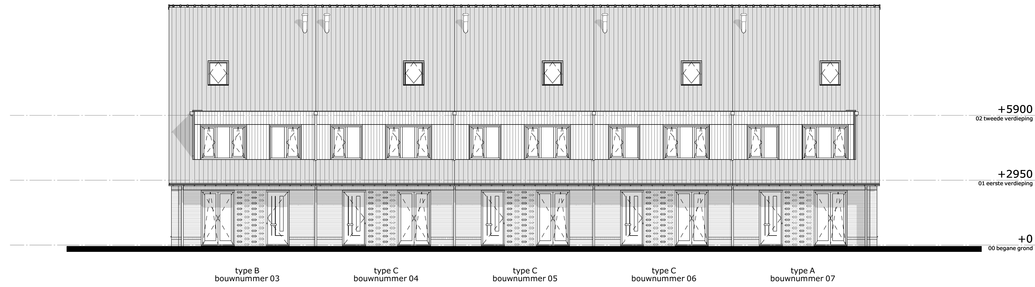
voorgevel
