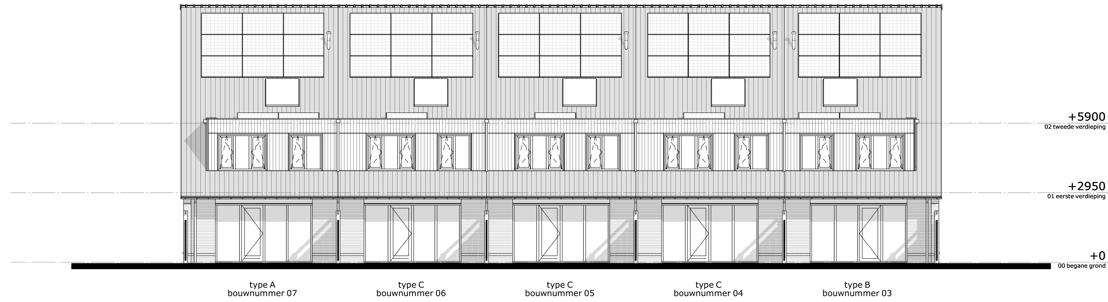
achtergevel
