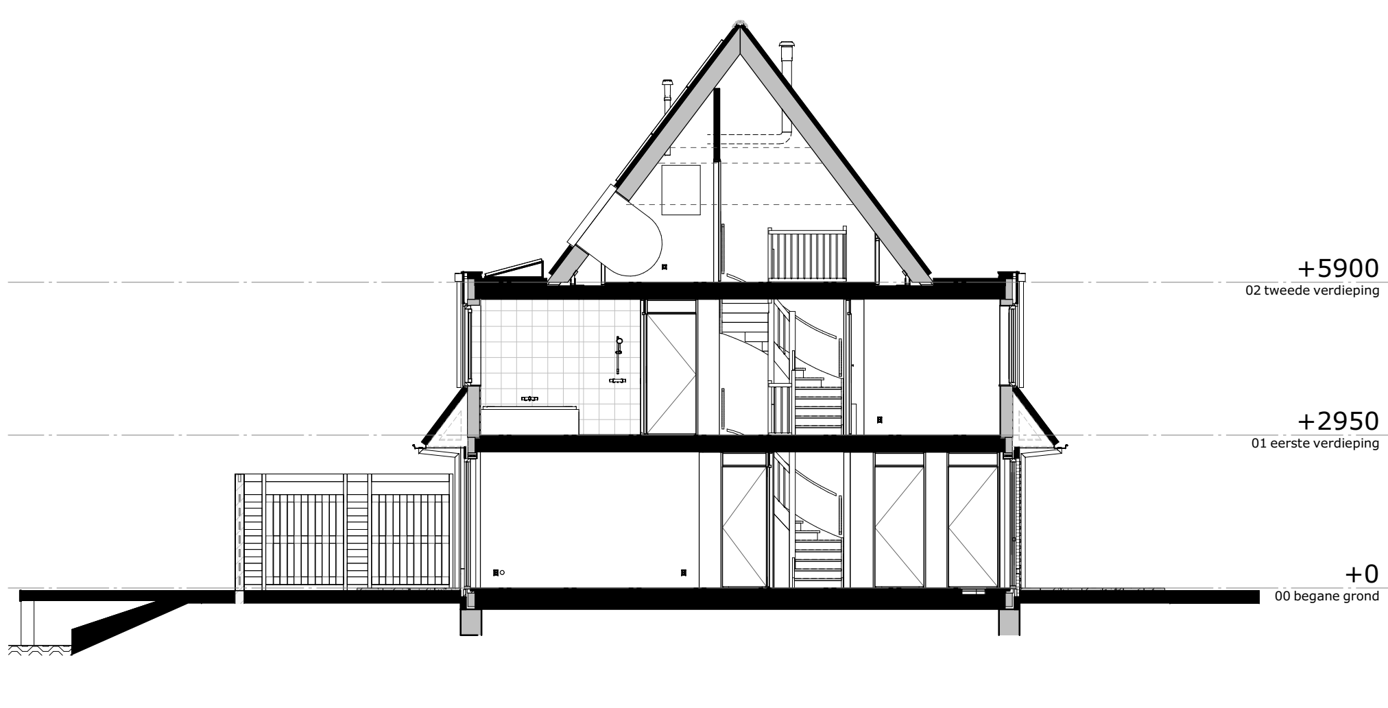
doorsnede A
