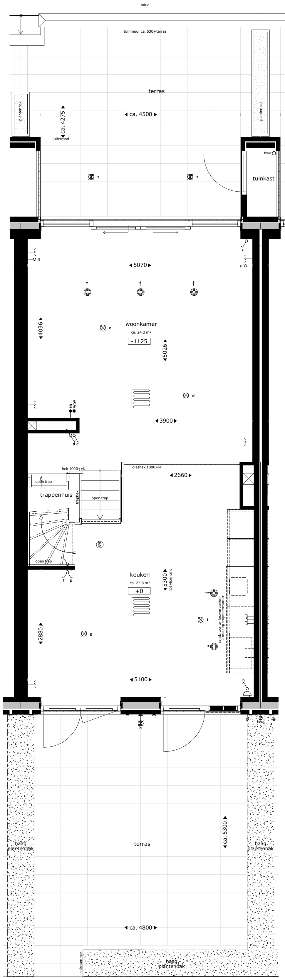
begane grond
