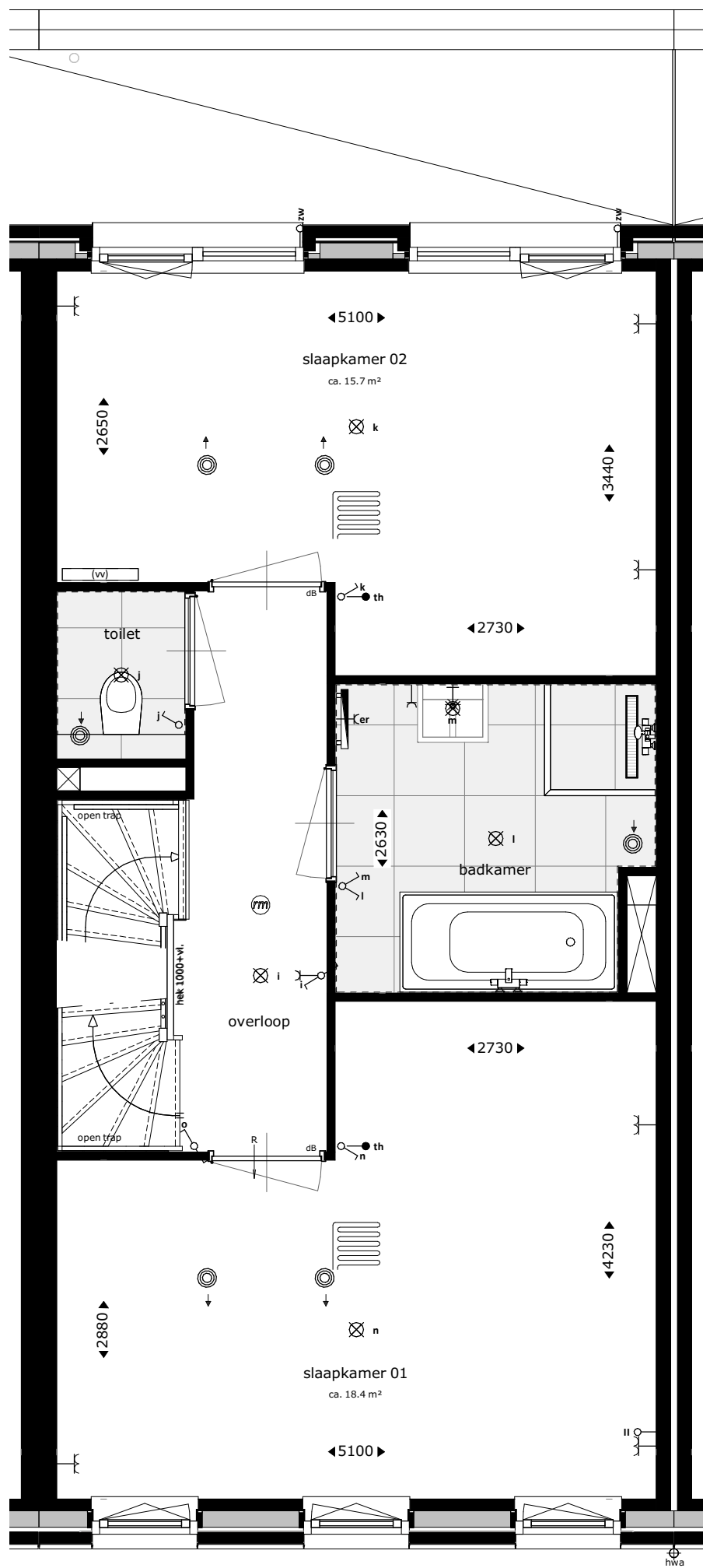
eerste verdieping
