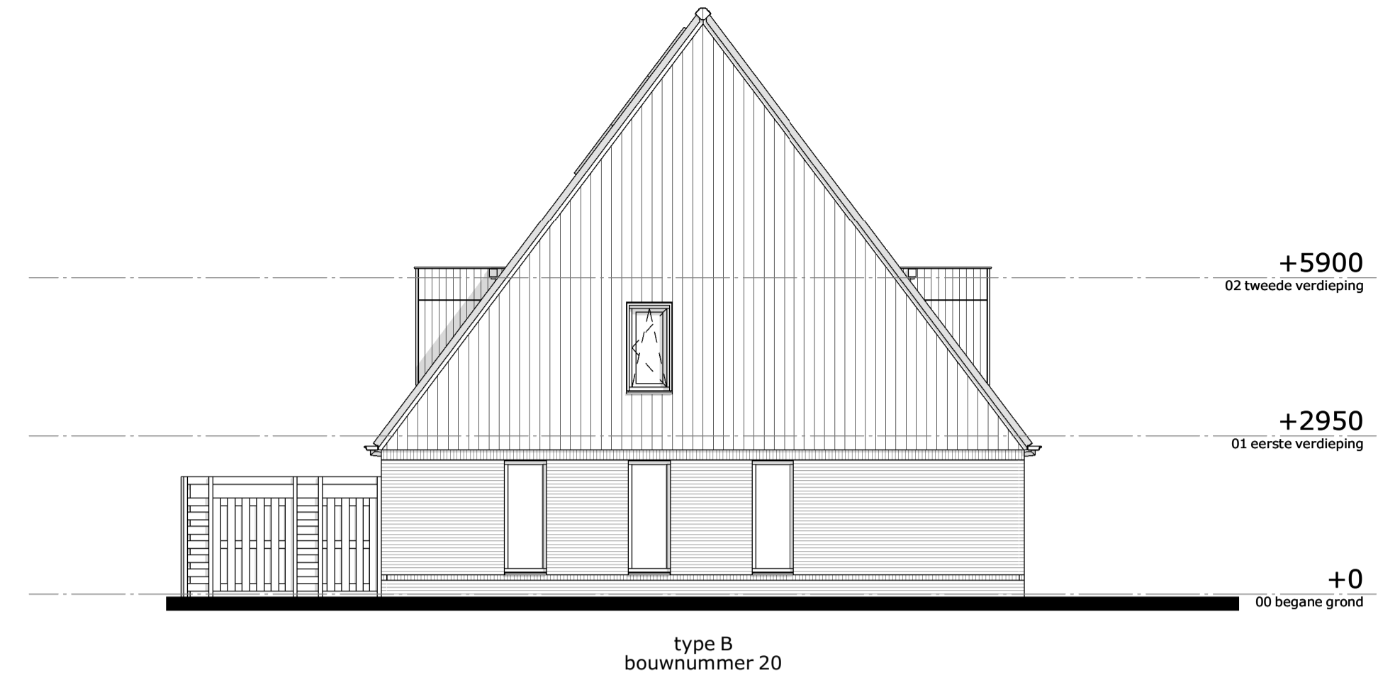
linker zijgevel
