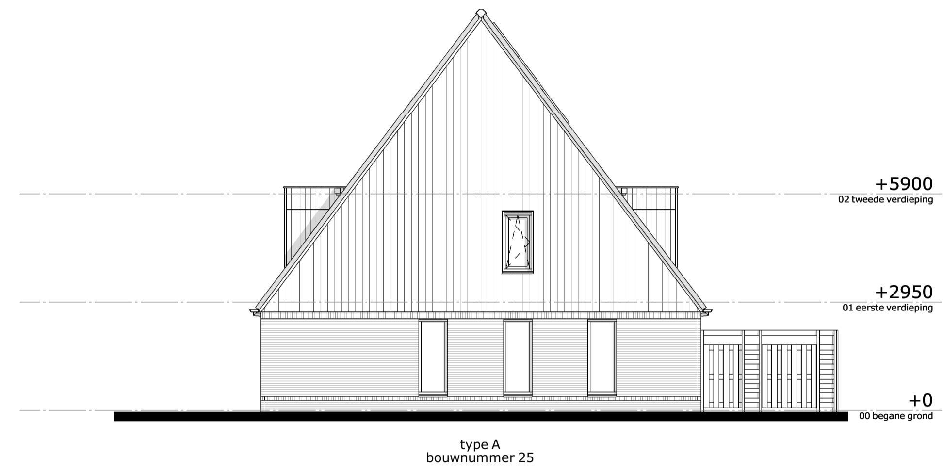
rechter zijgevel
