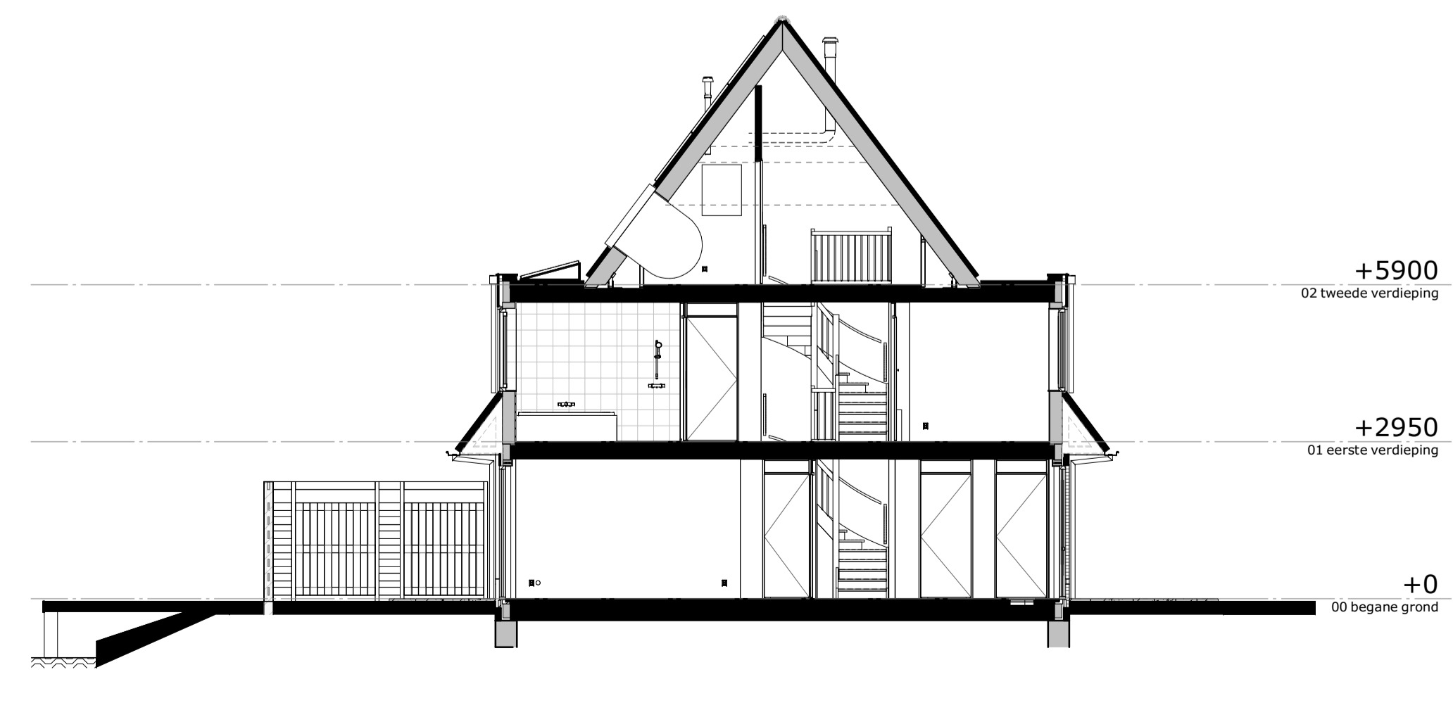
doorsnede A
